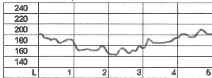
5 km:n latuprofiili
